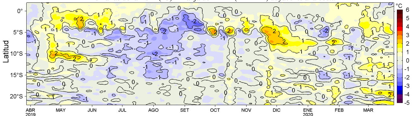
Figura 4. Variación promedio de las anomalías de la temperatura superficial del mar (TSM, °C) para una franja de 60 mn (~111 km) adyacente al litoral peruano para los últimos doce meses al 26 de marzo de 2020. Datos: OSTIA-UKMO-L4-GLOB-v2.0 (UK Met. Office, 2012; Donlon et al, 2012) disponible en https://podaac.jpl.nasa.gov/dataset/OSTIA-UKMO-L4-GLOB-v2.0 . Las anomalías se calcularon con respecto al periodo 2007-2016. Procesamiento: LHF/AFIOF/DGIOCC/IMARPE.
