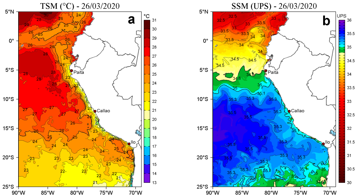
Figura 2. a) Temperatura superficial del mar (TSM, °C) y b) Salinidad superficial del mar (SSM, UPS), para el 26 de marzo de 2020. Datos: OSTIA-UKMO-L4-GLOB-v2.0 (UK Met Office, 2012; Donlon et al, 2012) disponible en https://podaac.jpl.nasa.gov/dataset/OSTIA-UKMO-L4-GLOB-v2.0 para (a) y Hybrid Coordinate Ocean Model v. GOF3.1 (HYCOM; Halliwell et al., 1998; 2000; Bleck, 2001) para (b). Procesamiento: LHF/AFIOF/DGIOCC/IMARPE.
