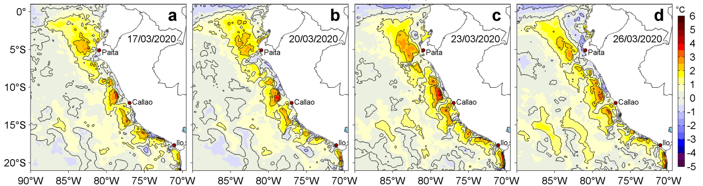
Figura 3. Anomalías de la temperatura superficial del mar (TSM, °C) para los días: a) 17, b) 20, c) 23 y d) 26 de marzo de 2020. Las anomalías se calcularon respecto de la climatología para el periodo 2007-2016. Datos: OSTIA-UKMO-L4-GLOB-v2.0 (UK Met Office, 2012; Donlon et al, 2012). Procesamiento: LHF/AFIOF/DGIOCC/IMARPE.
