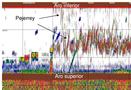
Figura 03 Ecograma con ecos de pejerrey ( Odontesthes bonariensis ) observados en la frecuencia de 120 kHz.
