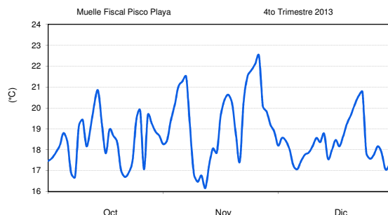
Fig. 8 Temperatura superficial del mar
