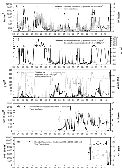
Figura 6. Parámetros comunitarios del bentos frente a Callao, 94 m. a) Densidad y N° de especies; b) biomasa de macrofauna y de nemátodos; c) biomasa de Thioploca spp. y porcentaje de vainas con tricoma; d) densidad y N° de taxones (0-1 cm) de la meiofauna metazoaria; e) densidad y N° de taxones (0-1cm) de foraminíferos bentónicos.
