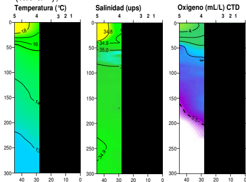
Figura. 3 Distribución vertical de: Temperatura, Salinidad y Oxígeno Perfil Hidrográfico Paita 1311 L/P Mi Marisol.
