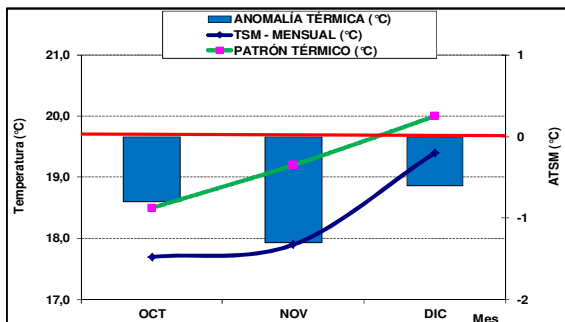
Figura 6. Variación de la temperatura y anomalía térmica durante los meses de octubre a diciembre del 2013 respecto al patrón
