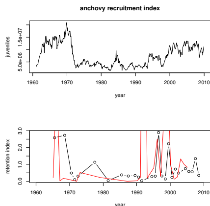
Figura 2. Panel superior: Serie de tiempo de reclutamiento de anchoveta entre el periodo 1961 y 2009. panel inferior: Serie de tiempo de la proporción entre larvas y huevos de anchoveta (línea negra corresponde a invierno y línea roja a verano).
