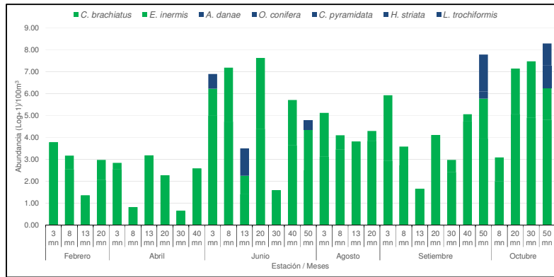
Figura 4. Indicadores de zooplancton en la EFC (Callao) durante el año 2013.
