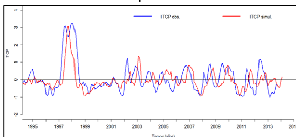
Figura 8. Pronóstico del ITCP mediante un modelo empírico, con datos actualizados hasta el mes de octubre del 2013.
