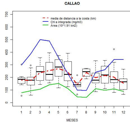
Figura 3. Ciclo estacional de: a) la distancia del frente de clorofila a la costa (1 mg/m 3 , rojo), b) clorofila integrada desde la distancia del frente de clorofila a la costa (azul) y c) área de la zona productiva (verde) para la zona de Callao.
