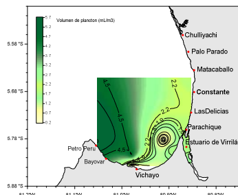
Figura 7. Distribución en superficie de los volúmenes de plancton (mL/m 3 ), en el estudio de la calidad marina en el Estuario de Virrila y Bahía de Sechura, octubre 2013
