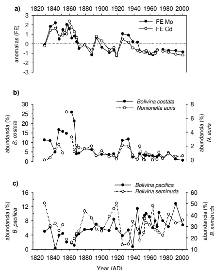
Figura 2. a) anomalías de los factores de enriquecimiento (FE) de Mo y Cd normalizadas por Al a lo largo del testigo B0405-13 (Callao 2004). Registros de la abundancia (%) de las especies de foraminíferos bentónicos consideradas indicadoras: b) de condiciones mayor sedimentación (material fresco, B. costata y N. auris ) y c) condiciones más oxigenadas ( B. pacífica ).
