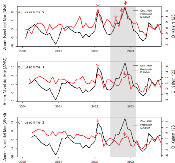
Figura 7. Variación temporal de la anomalía del nivel del mar observada (línea negra) y la predicción de la onda Kelvin (línea roja) (contribución conjunta de los modos 1, 2 y 3 a las anomalías del nivel mar en cm) sin el forzante de vientos en el punto grilla 0°N 90°W con a) 1 mes, b) 2 meses y c) 3 meses de anticipación durante 2000-2003. Periodo del evento El Niño 2002-03 (área gris) según el Índice ONI (NOAA, 2004).
