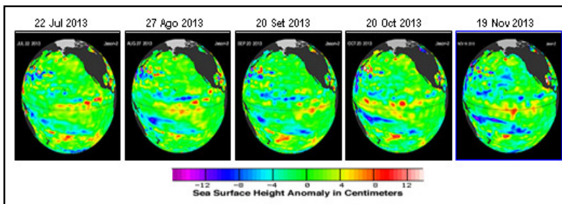
Fig. 2. Evolución mensual de la Anomalia de la Altura Superficial del Nivel del Mar en el Pacífico ecuatorial tropical del 22 julio 2013 al 19 noviembre 2013.
