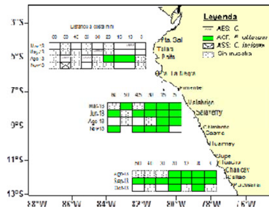
Figura 5. Indicadores Biológicos de masas de agua (fitoplancton) en la ECF Callao 1310 y los Perfiles Hidrográficos Paita y Chicama 1311
