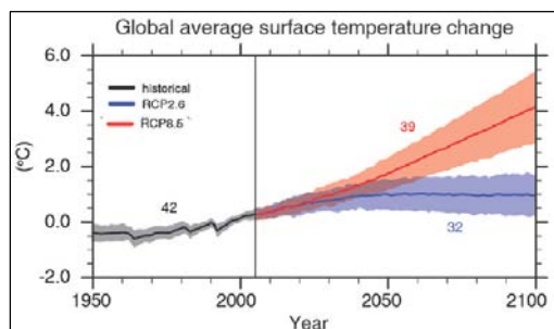
Figura 1. Cambio de la temperatura superficial promedio global según los escenarios RCP2.6 y RCP8.5 (Fuente: IPCC).
