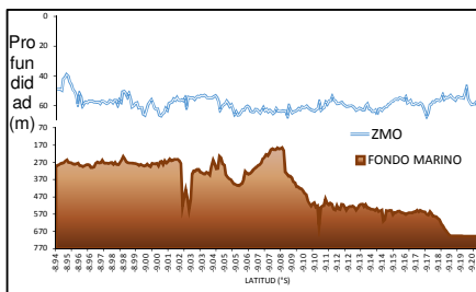
Fig. 01 - Límite superior de la ZMO detectada acústicamente
