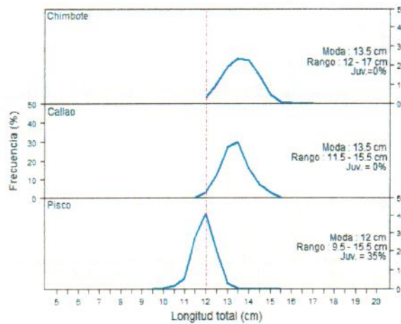
Estructura de tallas de la anchoveta proveniente de la flota artesanal y/o menor escala
