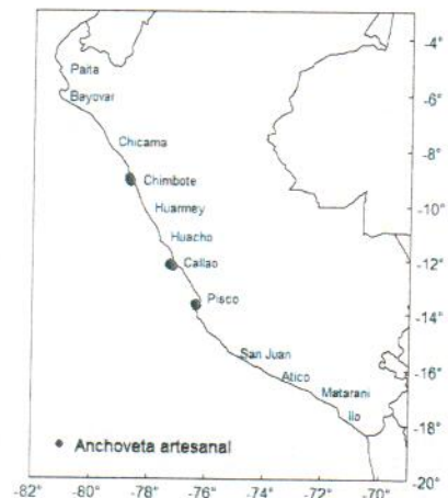
Zonas de pesca de anchoveta
