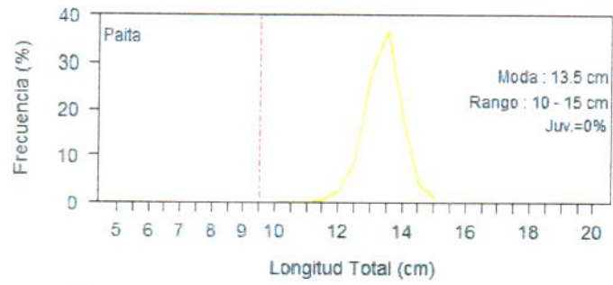
Estructura de tallas de samasa proveniente de la flota artesanal y/o menor escala
