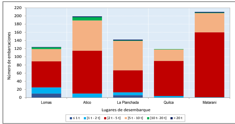
Estructura de la flota pesquera artesanal operativa según Capacidad de Bodega (t), Arequipa-Nov 2015.
