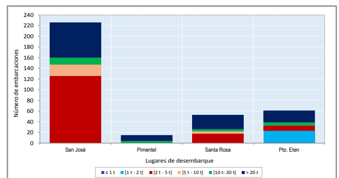
Estructura de la flota pesquera artesanal operativa según Capacidad de Bodega (t), Lambayeque-Nov 2015.
