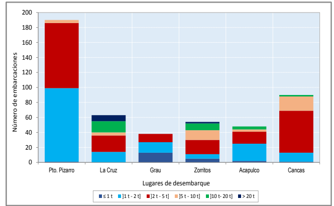
Estructura de la flota pesquera artesanal operativa según Capacidad de Bodega (t), Tumbes-Nov 2015.
