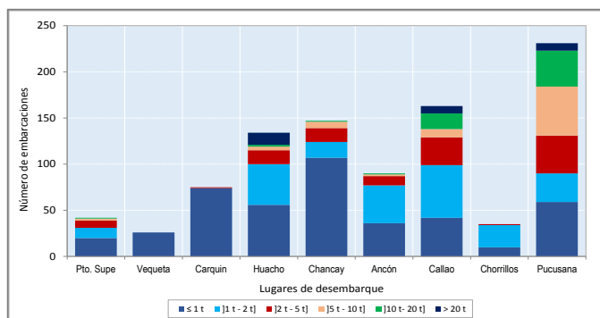
Estructura de la flota pesquera artesanal operativa según Capacidad de Bodega (t), Lima-Nov 2015.
