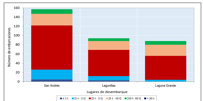
Estructura de la flota pesquera artesanal operativa según Capacidad de Bodega (t), Ica-Nov 2015.
