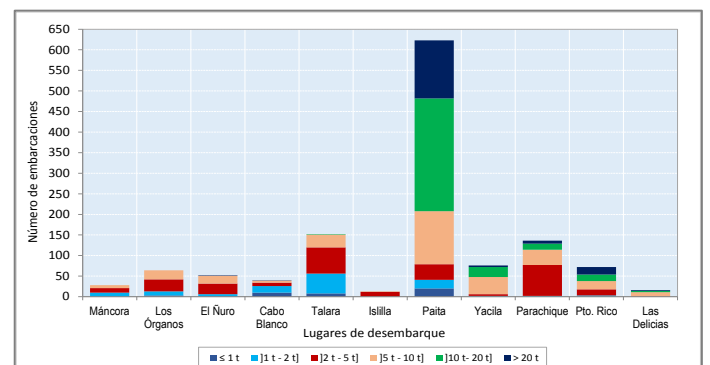
Estructura de la flota pesquera artesanal operativa según Capacidad de Bodega (t), Piura-Nov 2015.
