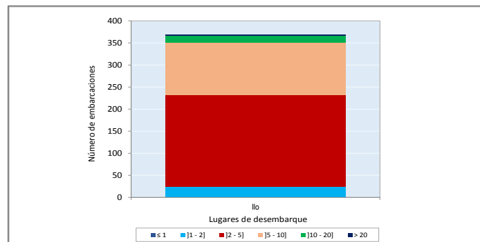
Estructura de la flota pesquera artesanal operativa según Capacidad de Bodega (t), Moquegua-Nov 2015.
