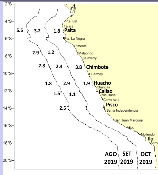
Figura 5. Valores promedio de contenido graso (CG) de anchoveta peruana Engraulis ringens por puertos durante agosto, setiembre y octubre del 2019.
