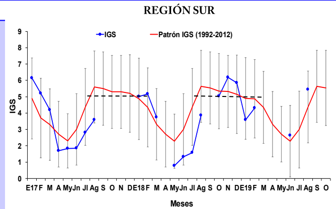
Figura 6. Índice gonadosomático (IGS) de anchoveta peruana Engraulis ringens de la región sur, desde enero 2017 a octubre del 2019 y el patrón 1992-2012.
