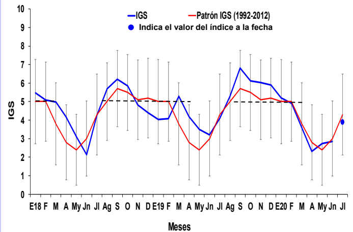
Figura 2. Índice gonadosomático (IGS) de anchoveta peruana Engraulis ringens de la región norte-centro, de enero 2018 a 15 julio 2020 con el patrón 1992-2012.
