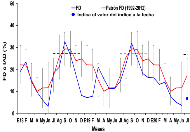
Figura 1. Fracción desovante o índice de actividad de desove (FD o IAD) de anchoveta peruana Engraulis ringens de la región norte-centro, de enero 2018 a 15 julio 2020 con el patrón 1992-2012 .
