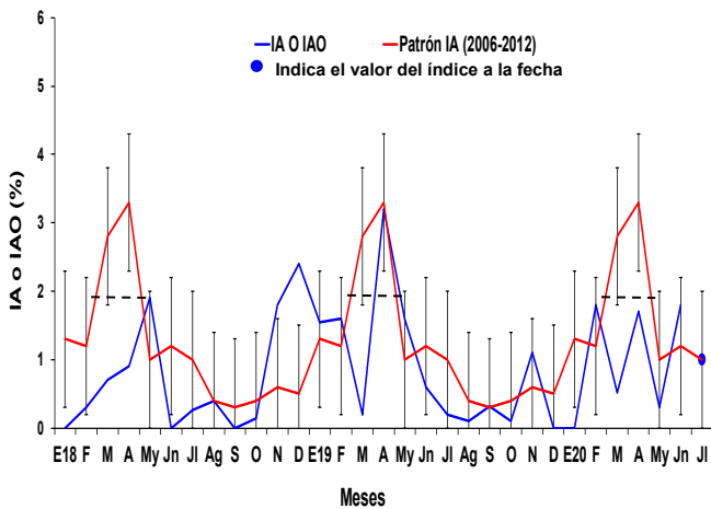
Figura 3. Índice de atresia o índice de atresia ovocitaria (IA o IAO) de anchoveta peruana Engraulis ringens de la región norte-centro, de enero 2018 a 15 julio 2020 con el patrón 2006-2012.
