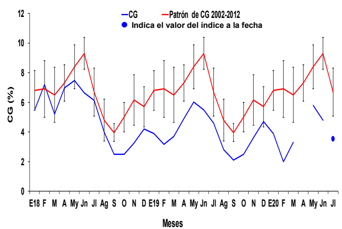
Figura 4. Contenido graso (CG) de anchoveta peruana Engraulis ringens de la región norte-centro, de enero 2018 a 15 julio 2020 con el patrón 2002-2012.
