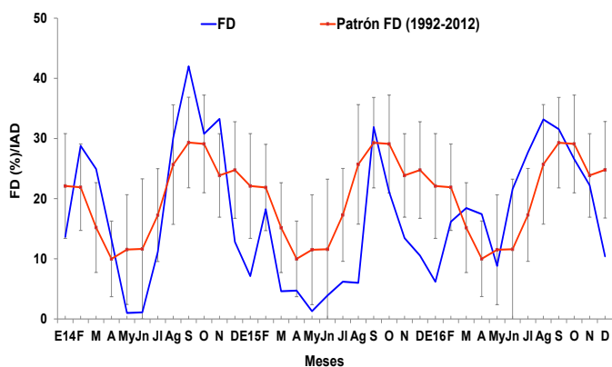
Figura 1. Fracción desovante o Índice de Actividad Desovante (FD/IAD) de anchoveta peruana Engraulis ringens de la región norte-centro de enero 2014 a diciembre 2016 con el patrón 1992-2012.
