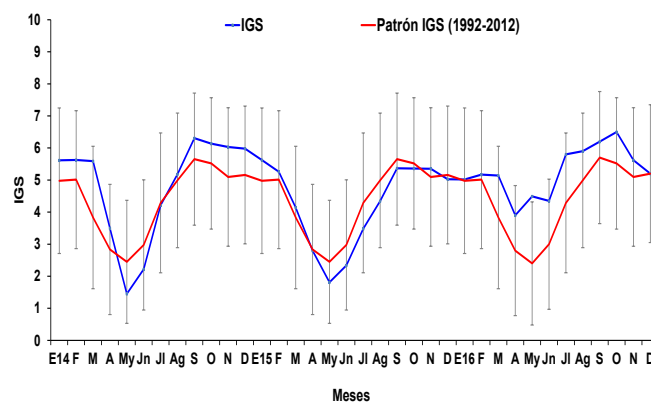
Figura 2. Índice gonadosomático (IGS) de anchoveta peruana Engraulis ringens de la región norte-centro de enero 2014 a diciembre 2016 con el patrón 1992-2012.
