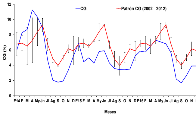
Figura 4. Contenido graso (CG) de anchoveta peruana Engraulis ringens de la región norte-centro de enero 2014 a diciembre 2016 con el patrón 2002-2012.
