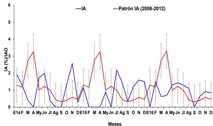
Figura 3. Índice de atresia o Índice de Atresia Ovocitaria (IA/IAO) de anchoveta peruana Engraulis ringens de la región norte-centro de enero 2014 a diciembre 2016 con el patrón 2006-2012.
