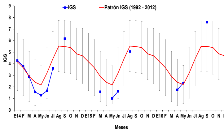
Figura 5. Índice gonadosomático (IGS) de anchoveta peruana Engraulis ringens del stock sur, desde enero 2014 hasta diciembre del 2016 y el patrón 1992-2012.
