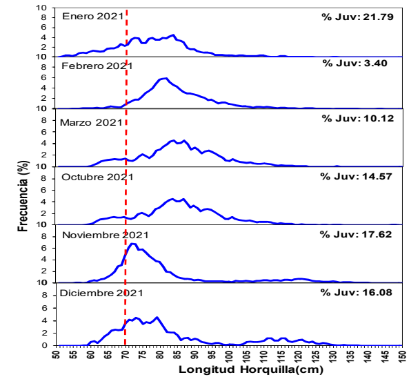
Estructura por Tallas de Perico (Enero a diciembre 2021)
