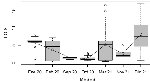
Biología reproductiva de Perico (Enero 2020 a Diciembre 2021)
