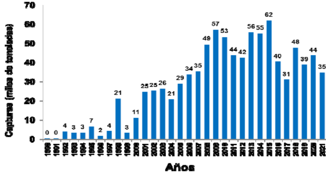
Capturas Anuales de Perico Total Perú (1990 - 2021)
