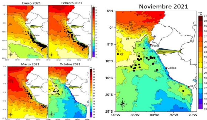
Áreas de Pesca de Perico (Enero a Noviembre 2021)
