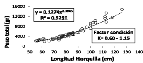
Biología reproductiva de Perico (Enero 2020 a Diciembre 2021)
