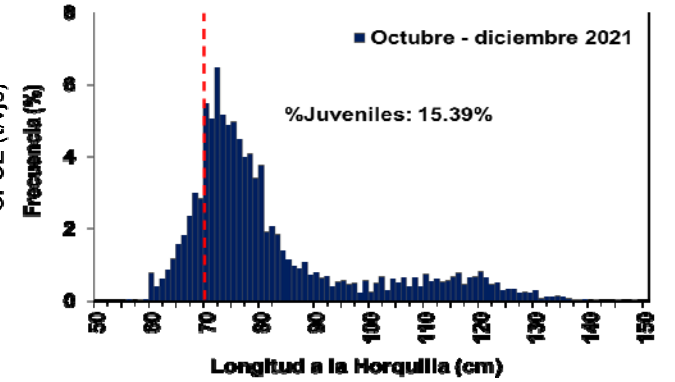
Estructura por Tallas de Perico (Octubre a diciembre 2021)
